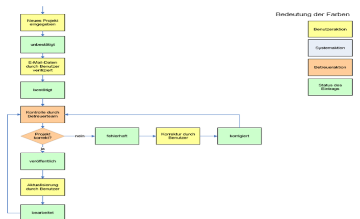
Zustandsflussdiagramm des Projekteintrags
