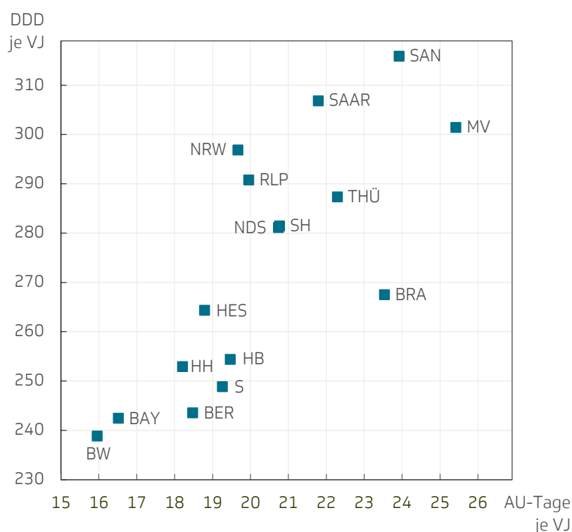
Abbildung 6 (standardisierte Werte zu 16 Bundesländern, Korrelationskoeffizient: r = 0,78 ; Korrelationskoeffizient bei Berücksichtigung von zwölf Bundesländern ohne die Stadtstaaten und Brandenburg: r = 0,85 )
